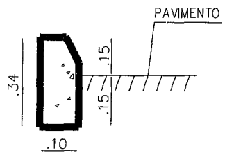
DETALHE MEIO-FIO EM CONCRETO SEM ESCALA
