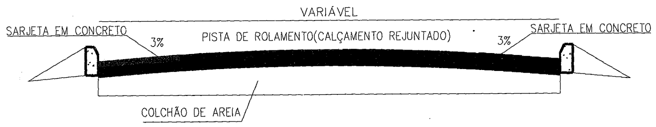
SEÇÃO TIPO SEM ESCALA
