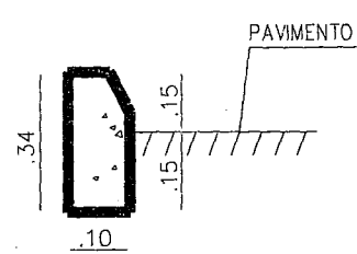
DETALHE MEIO-FIO EM CONCRETO SEM ESCALA
