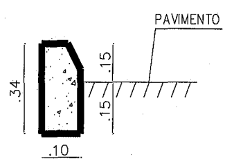
DETALHE MEIO-FIO EM CONCRETO SEM ESCALA
