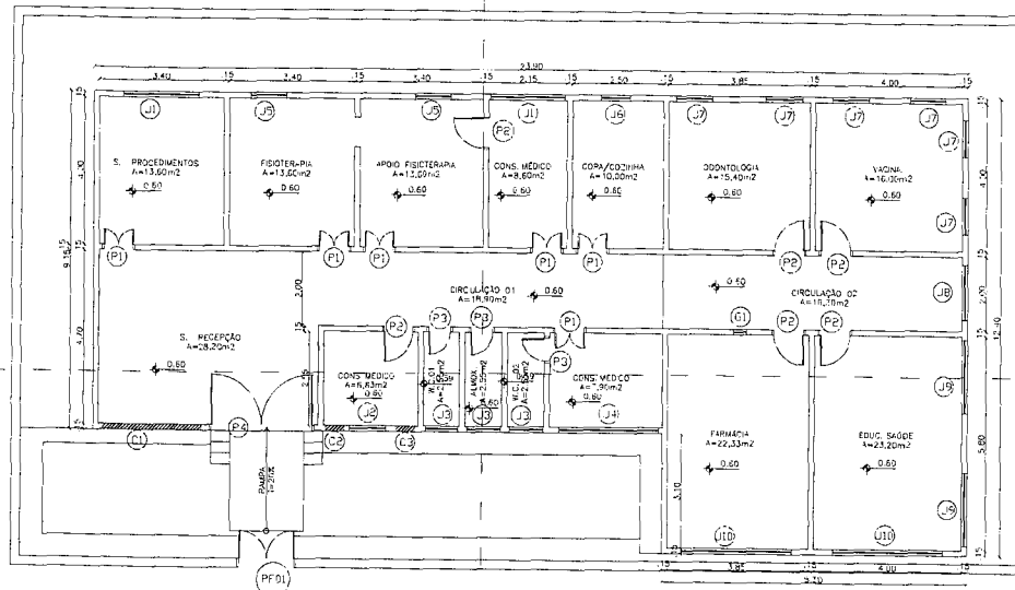
PLANTA BAIXA EXISTENTE esc. 1:75
