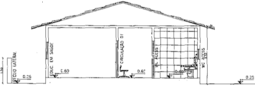
CORTE BB esc. 1:75
