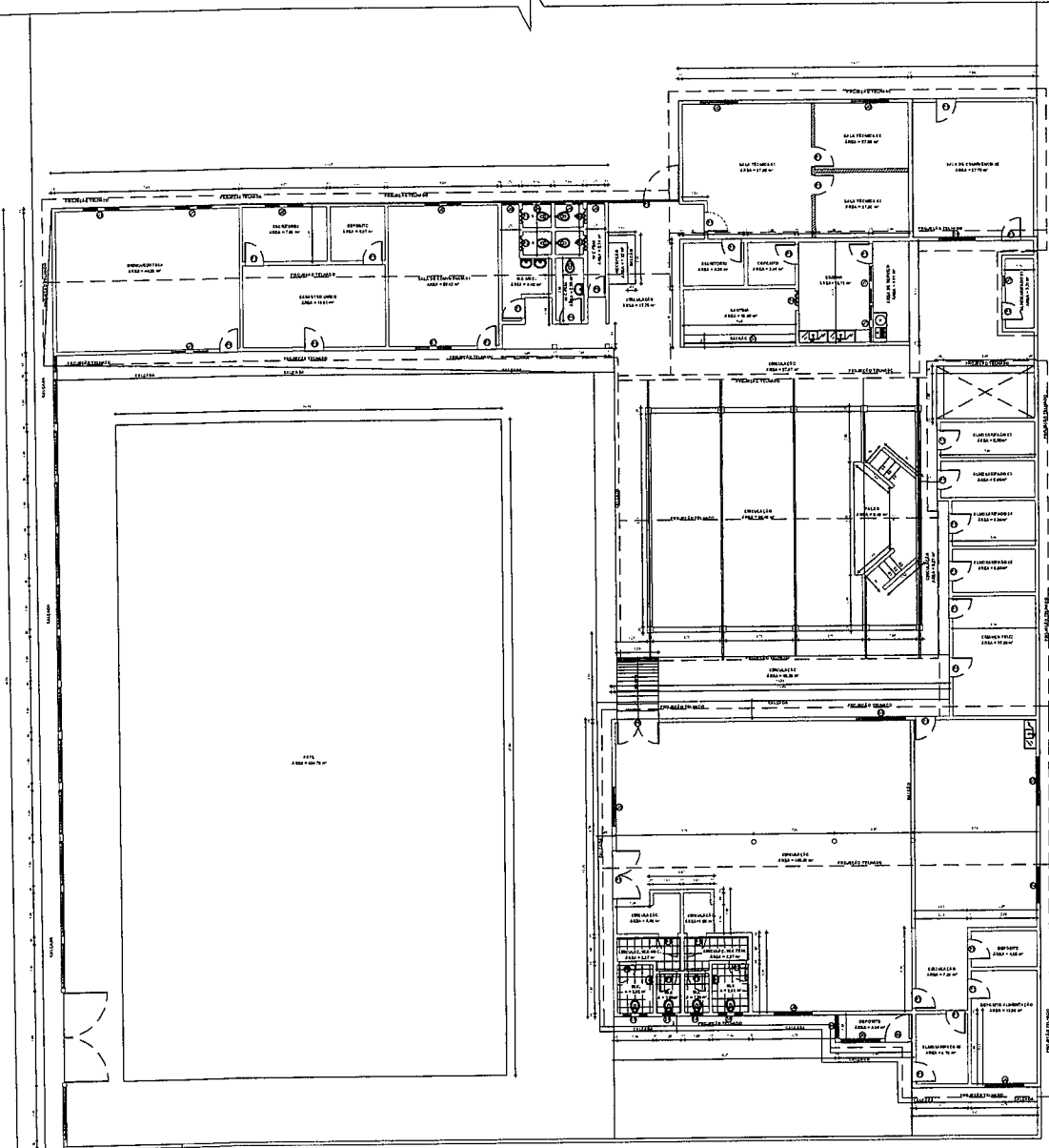
PLANTA BAIXA esc 1:100
